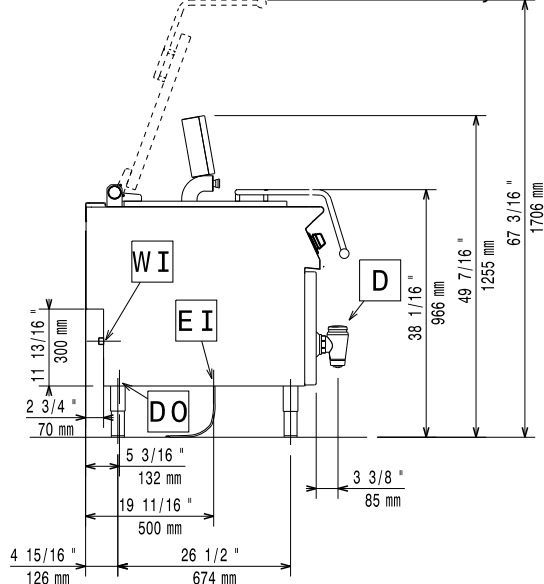
Zij aanzicht
